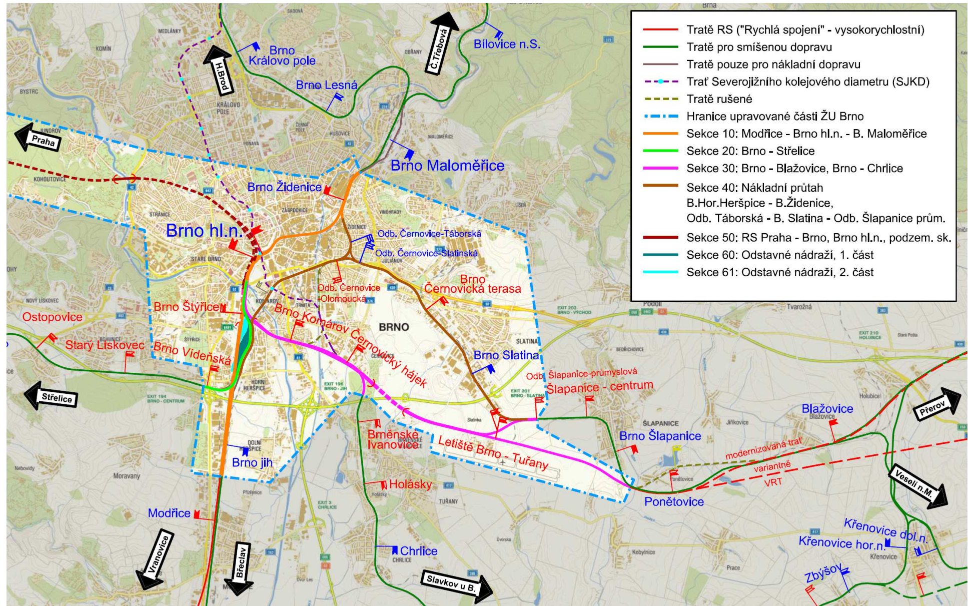
Obr. 2 Členění železničního uzlu Brno stavby
