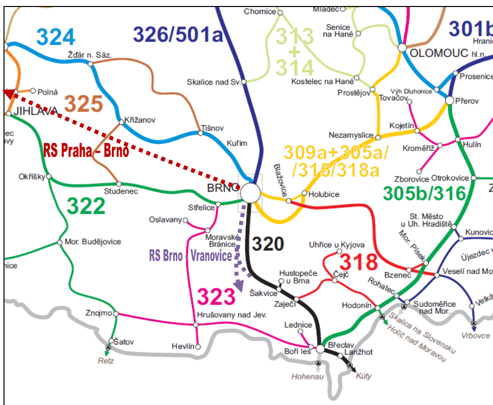
Obr. 1 Schéma tratí v okolí železničního uzlu Brno
